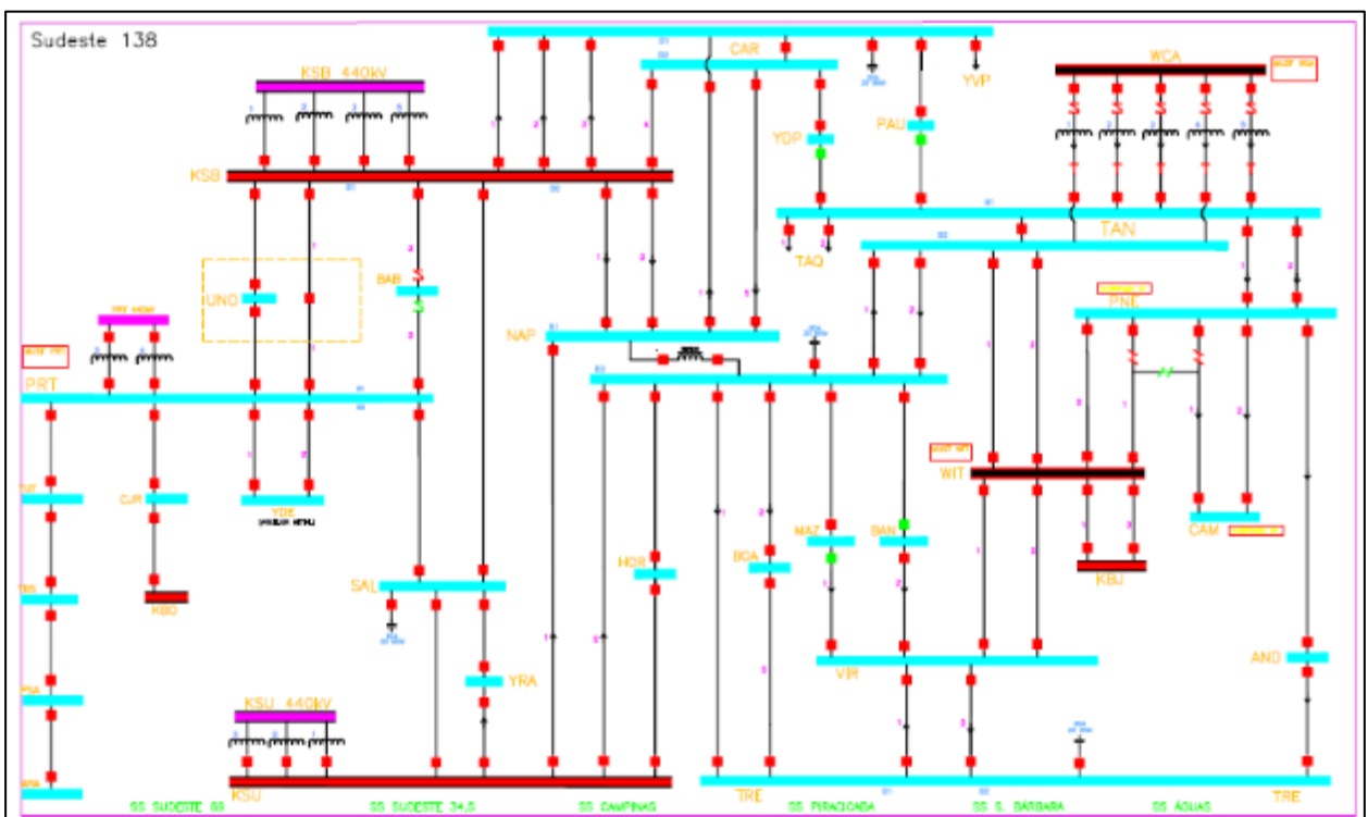
Figura 7 - Diagrama Unifilar de Subtransmissão da regional SUDESTE
