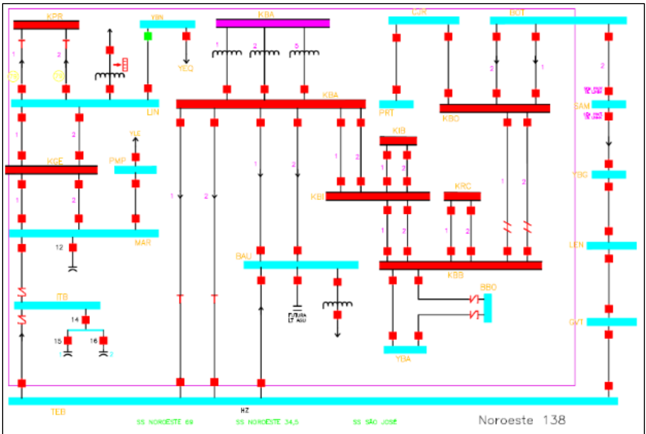
Figura 6 - Diagrama Unifilar de 138kV da Subtransmissão da regional NOROESTE
